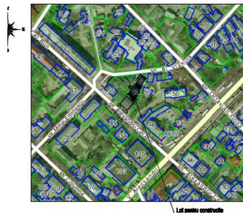
Plan de situație, Sc. 1:2000
